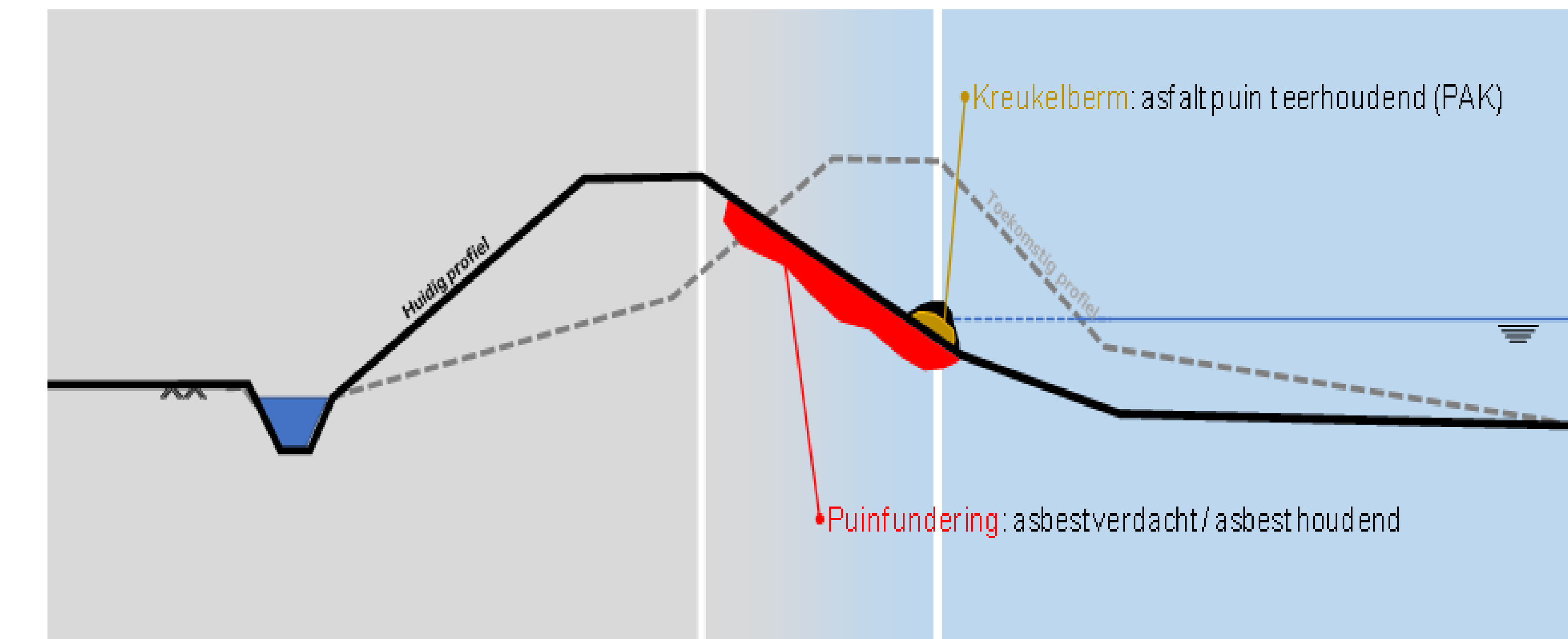
Locaties asbest en asfalt en de wijze van integreren in de nieuwe dijk
