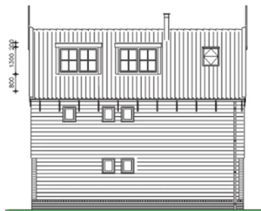
zijgevel. noordoost
