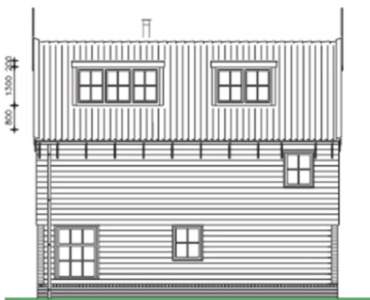
zijgevel. zuidwest
