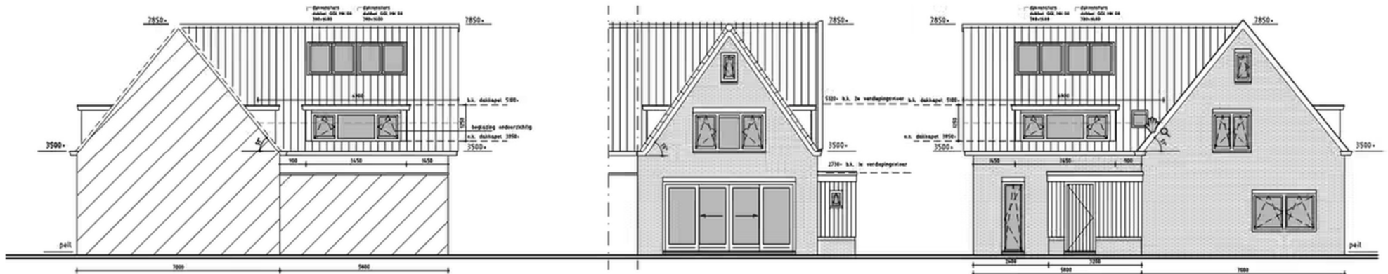
Rechter Zijgevel (gewijzigd)
