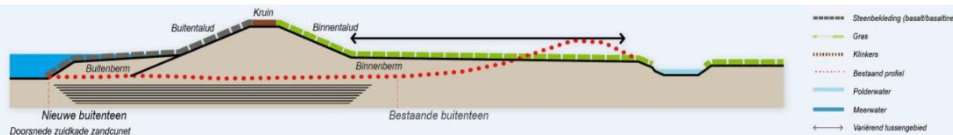
Figuur 2.6 Zuidkade maximaal profiel
