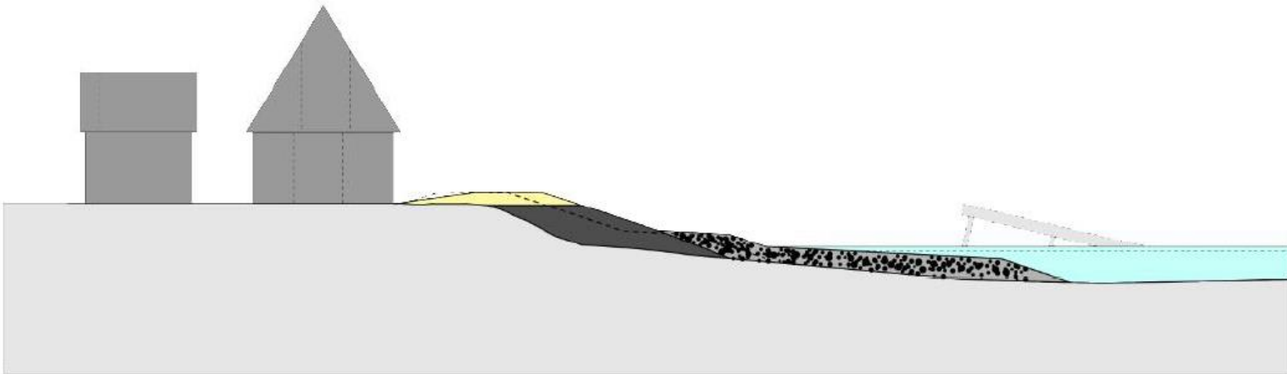
Figuur 2.9 Versterking bij de Rozewerf in dwarsprofiel
