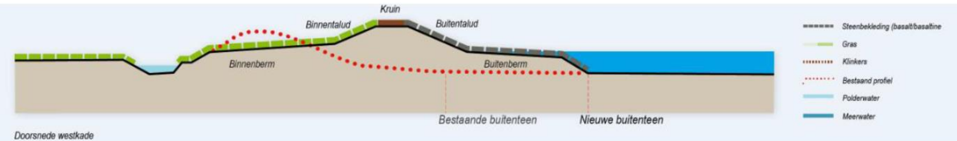
Figuur 2.3 Doorsnede Westkade
