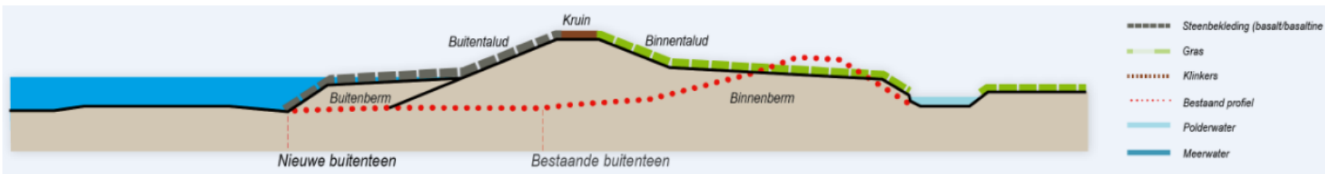
Figuur 2.5 Dwarsprofiel Zuidkade, compact profiel
