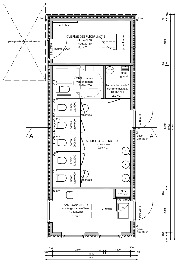
BEGANE GROND
