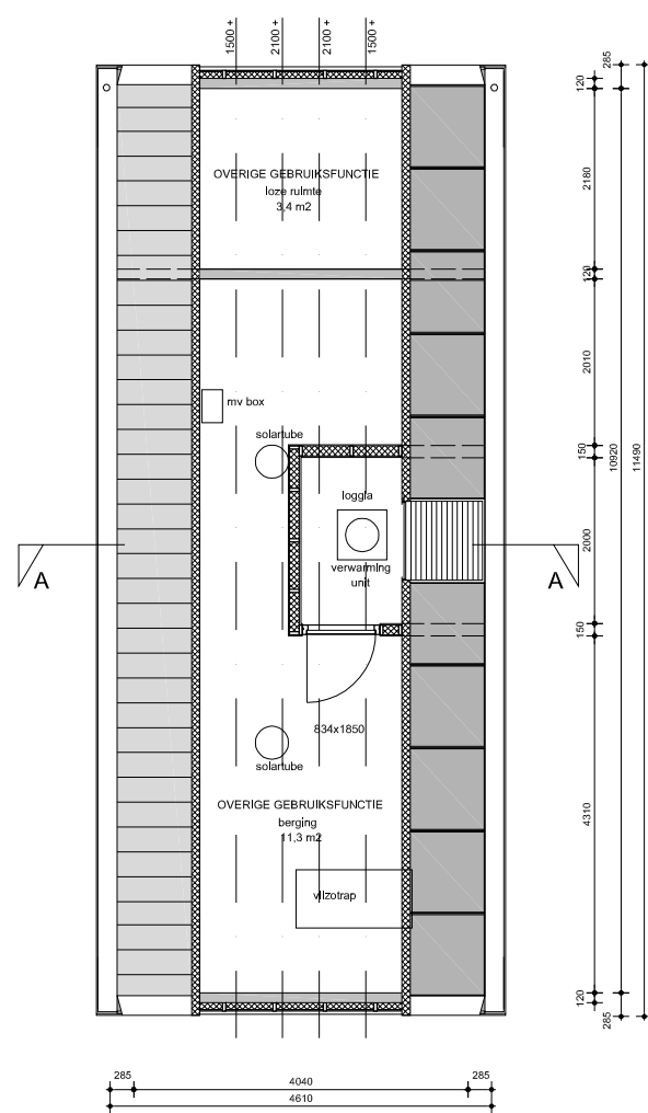
1E VERDIEPING
