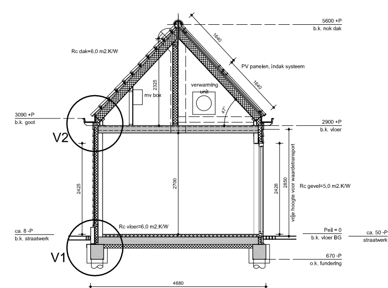
DOORSNEDE A-A
